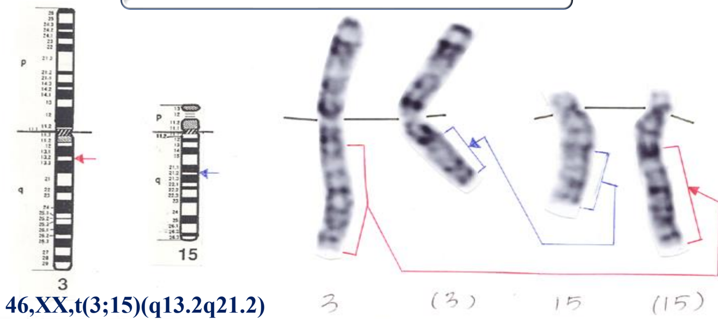
图3 染色体均衡型转座
